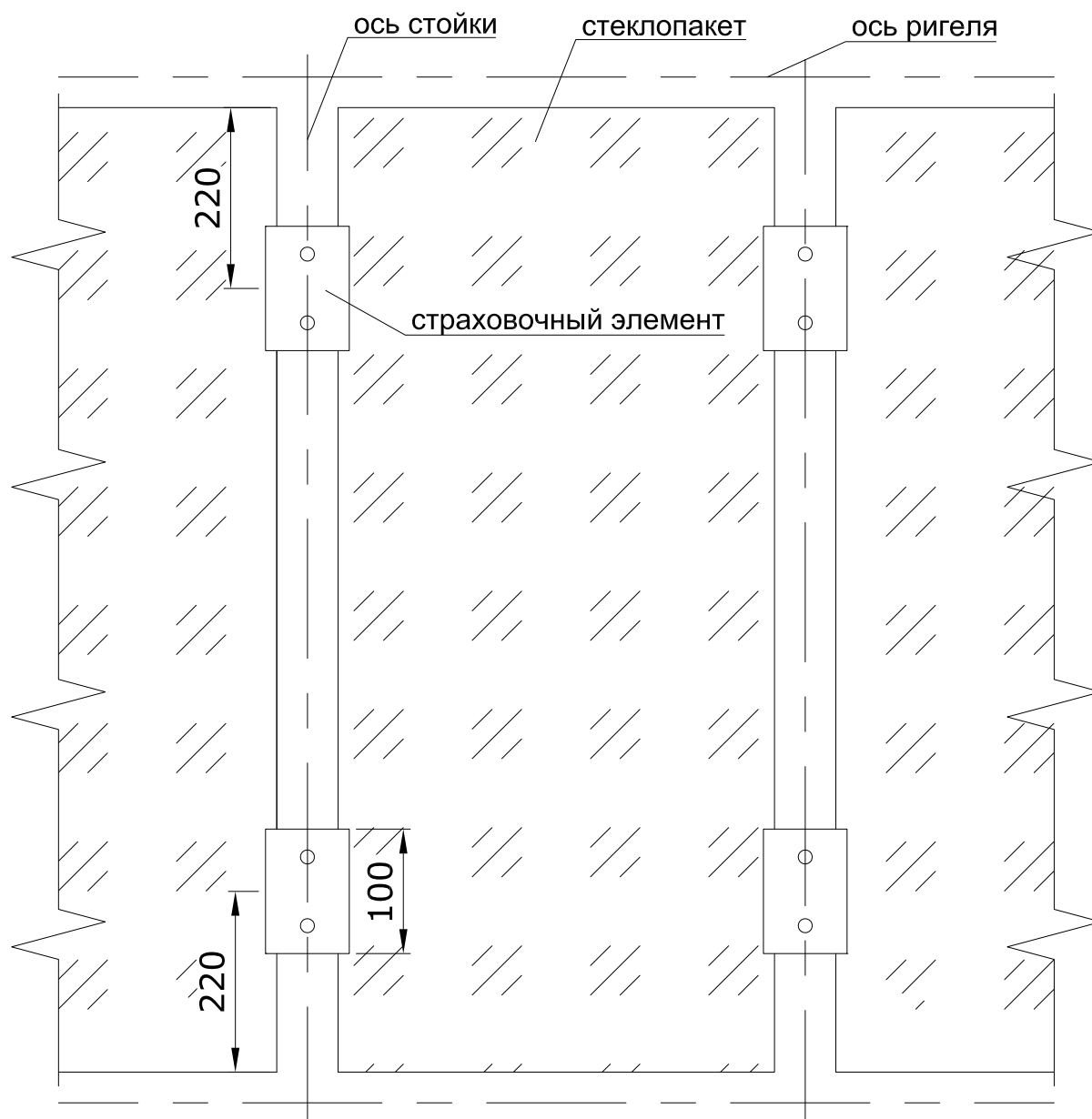
элементы страховки стеклопакета.
