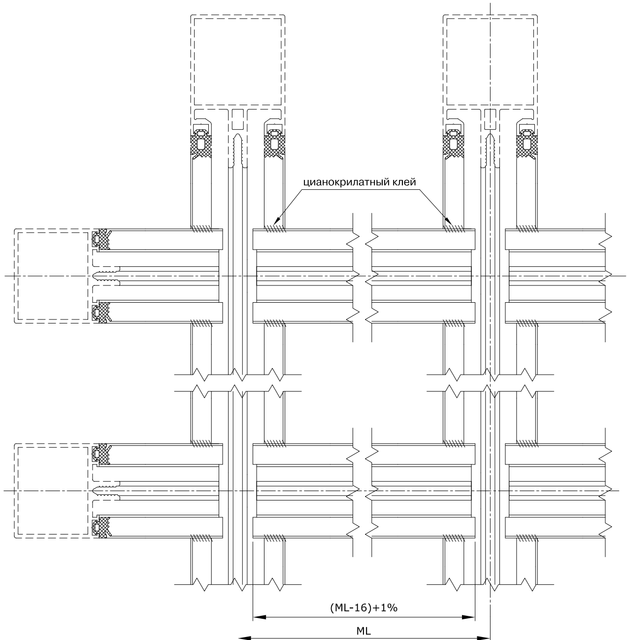
Схема установки уплотнителей
