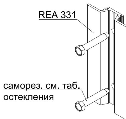
элементы страховки стеклопакета.
