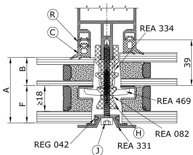
Сечение по стойке
